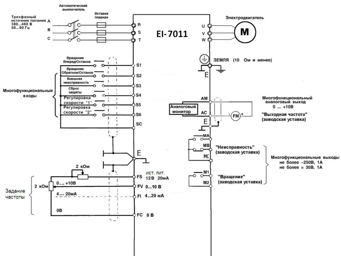
Рис. 9. Схема подсоединения.
